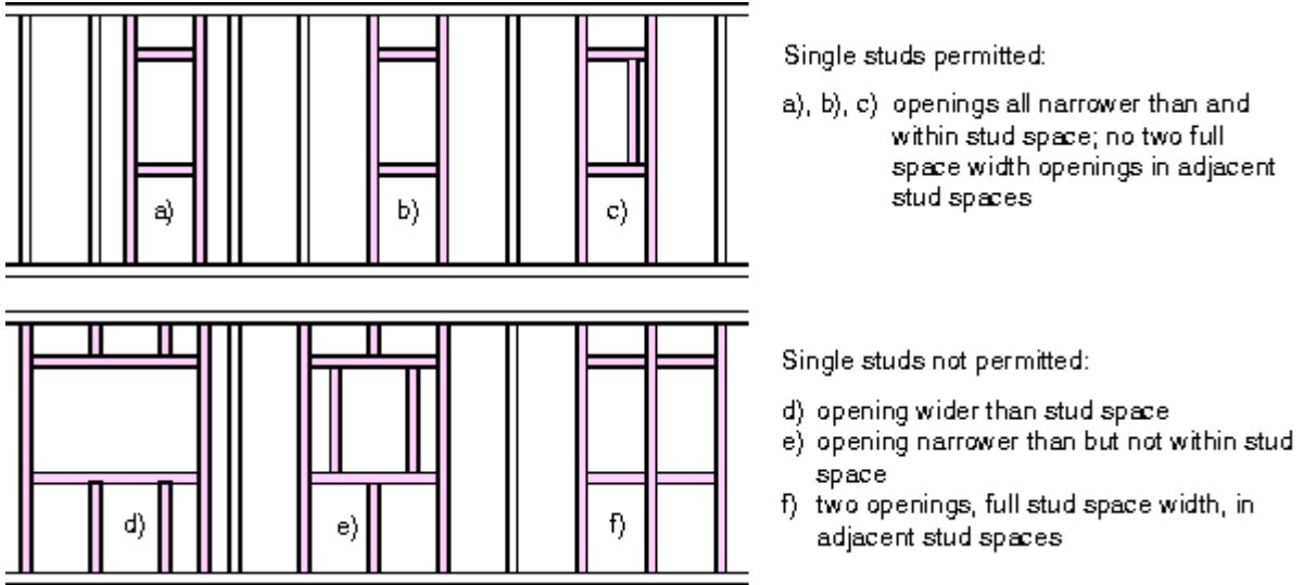
Figure A-9.23.10.6.(3)-B
