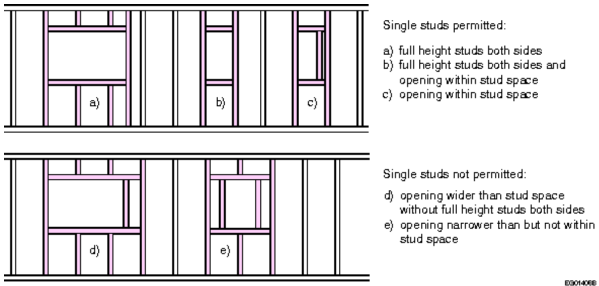
Figure A-9.23.10.6.(3)-A
