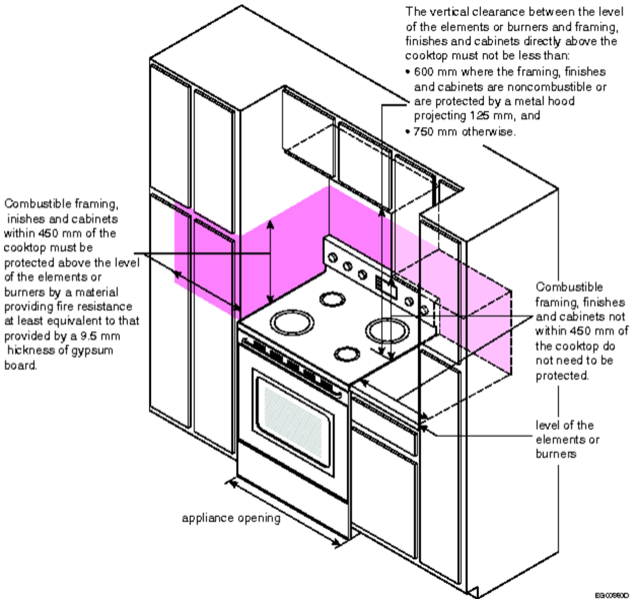
Figure A-9.10.22.
