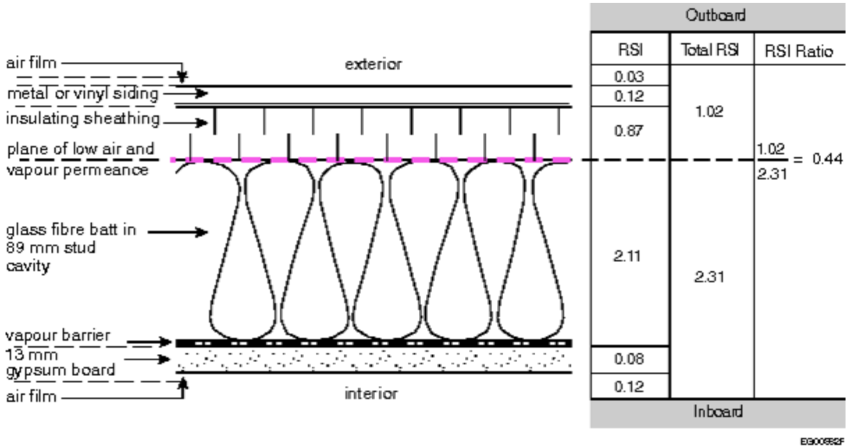
Figure A-9.25.5.2.
