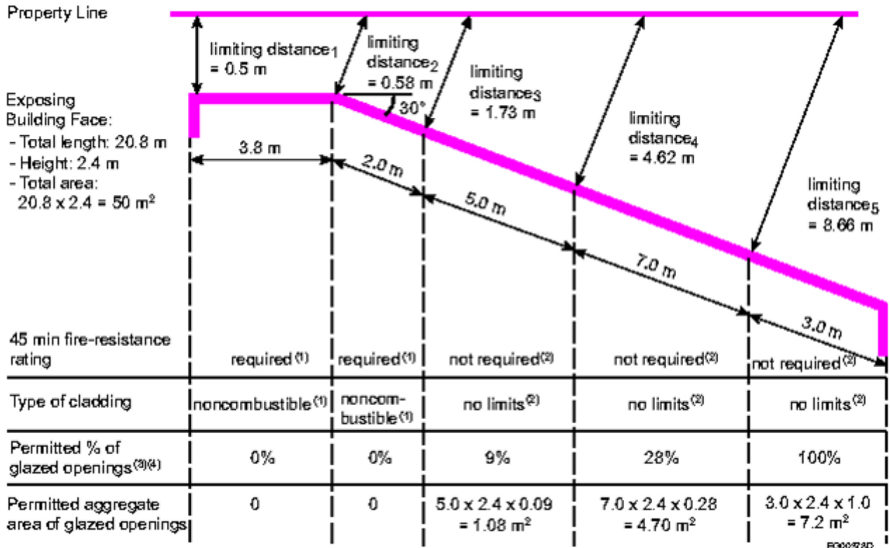
Figure A-9.10.15.4.(2)-B
