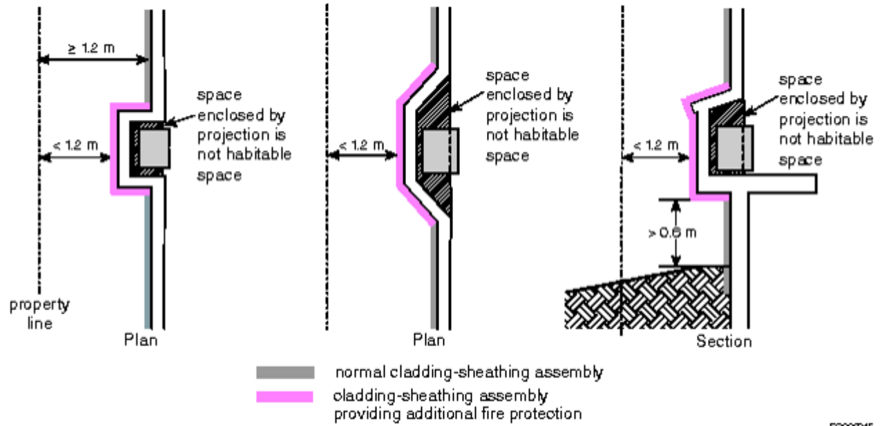
Figure A-9.10.14.5.(8)
