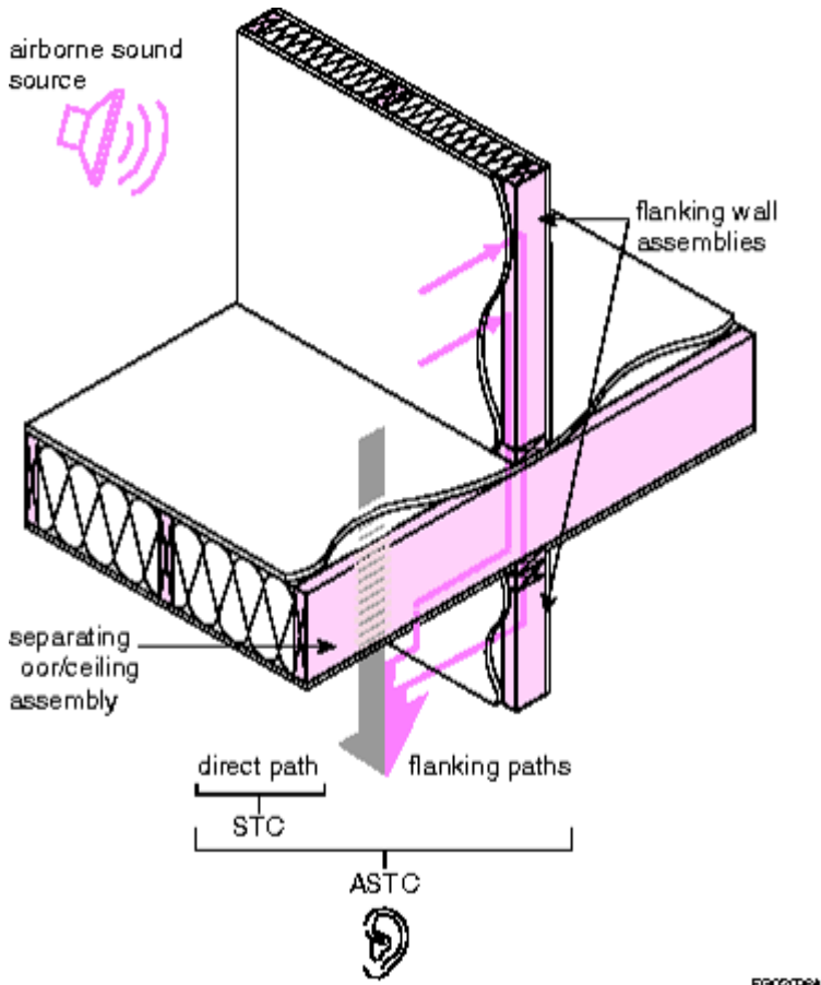
Figure A-9.11.-B
