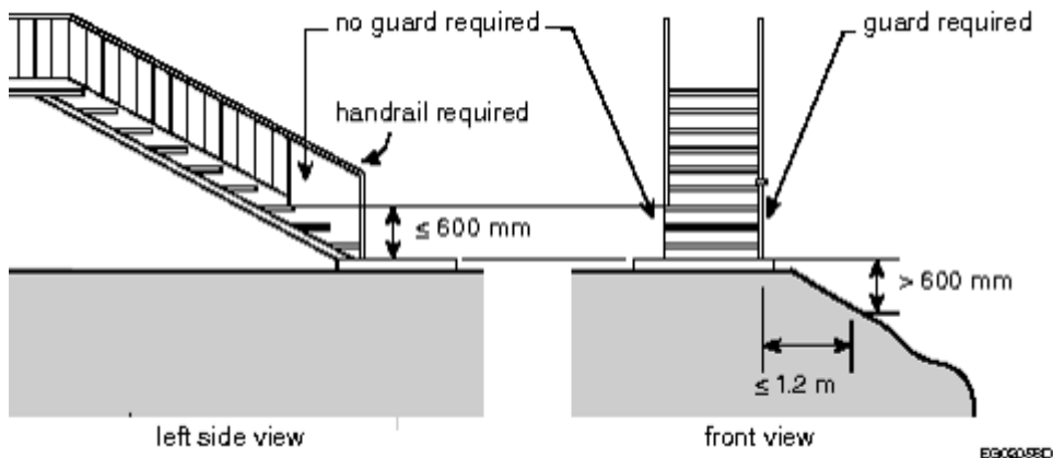
Figure A-9.8.8.1.
