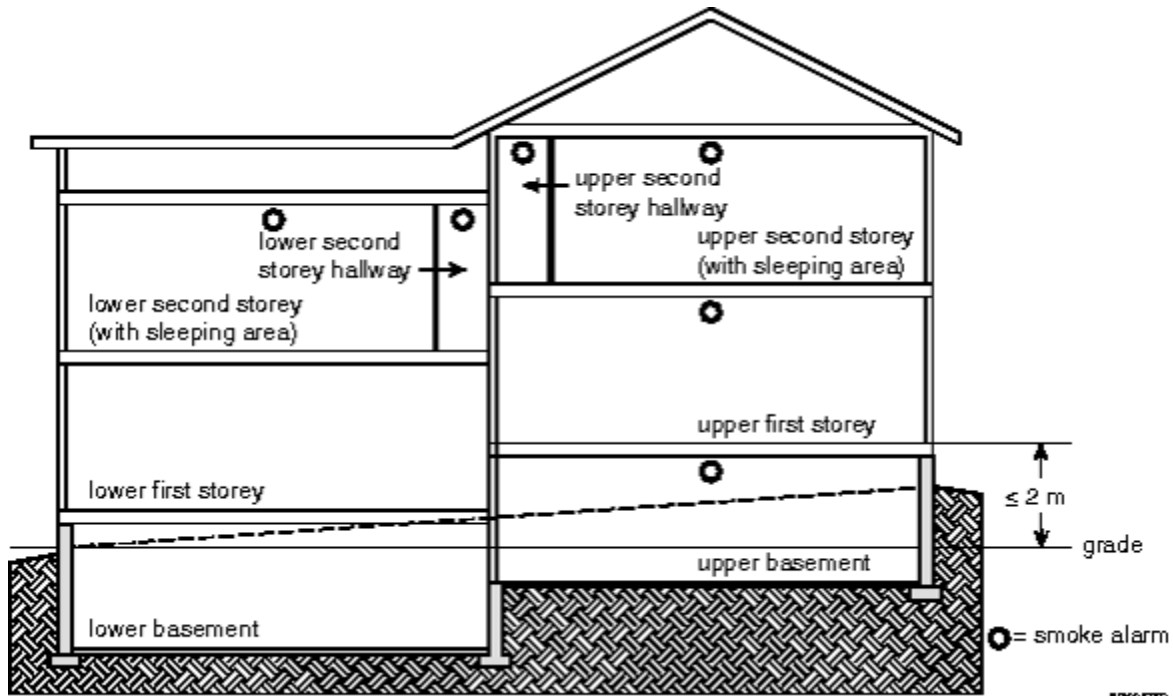
Figure A-9.10.19.3.(1)
