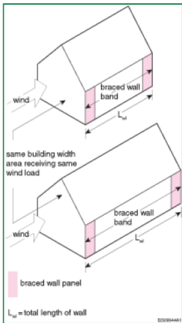
Figure A-9.23.13.7.(3)-A
