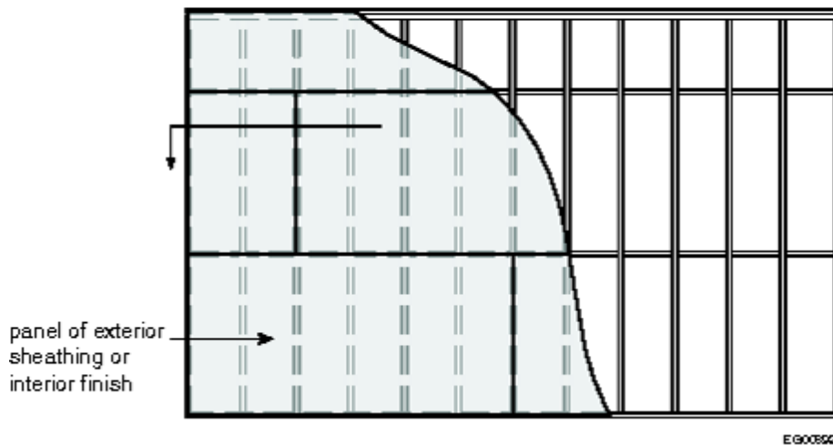
Figure A-9.10.3.1.-G
