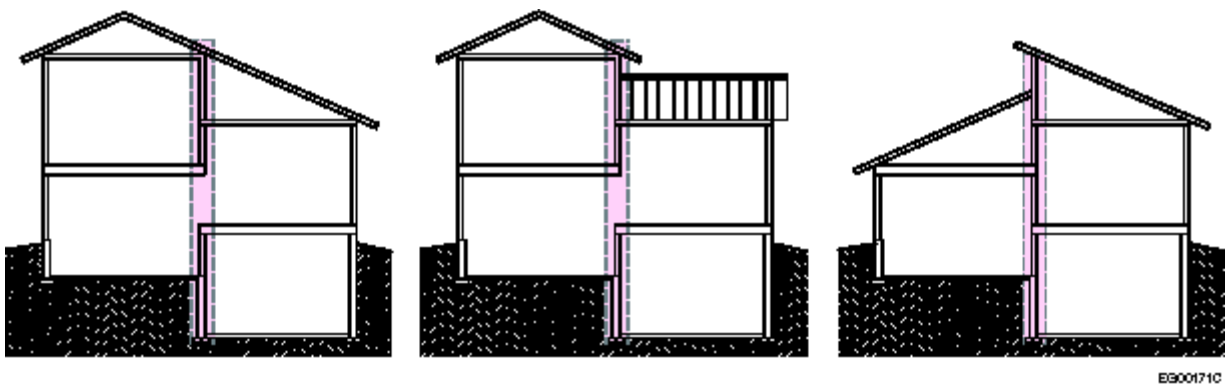
Figure A-9.23.13.4.-C
