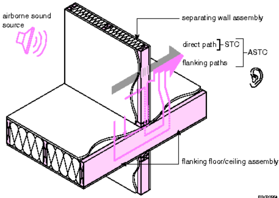
Figure A-9.11.-A
